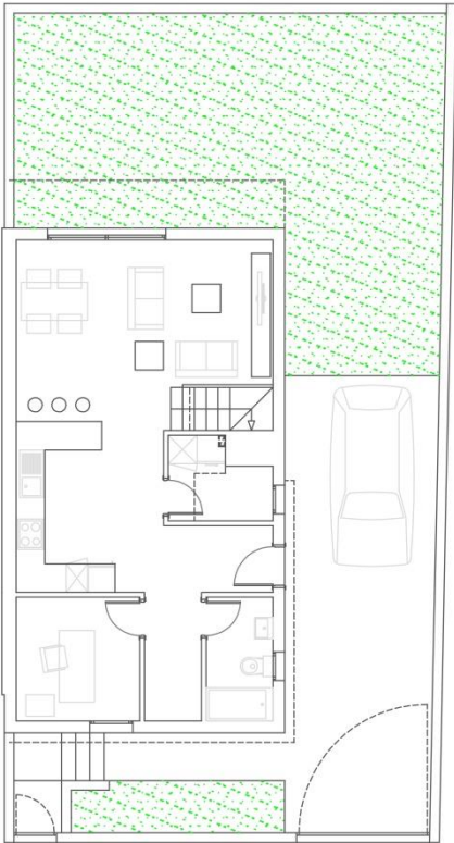
PLANTA BAJA
