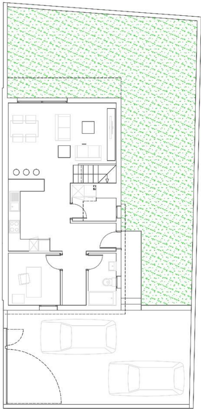
PLANTA BAJA
